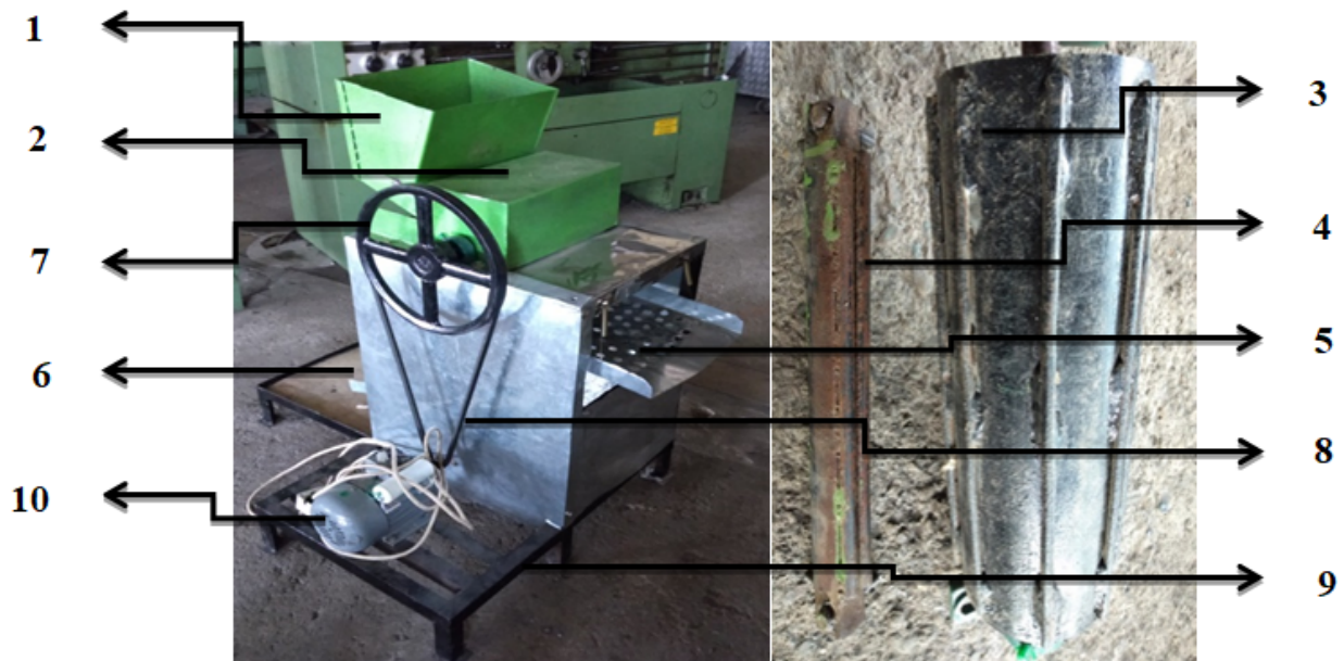
Gambar 11 . Mesin pengupas kulit kacang tanah dengan tipe silinder horizontal
